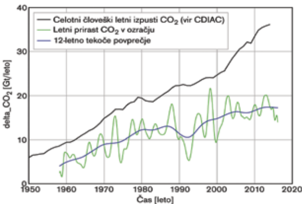
Diagram 5 kaže primerjavo letnih prirastkov \text{CO}_2 v človeških izpustih s tistimi v ozračju.
